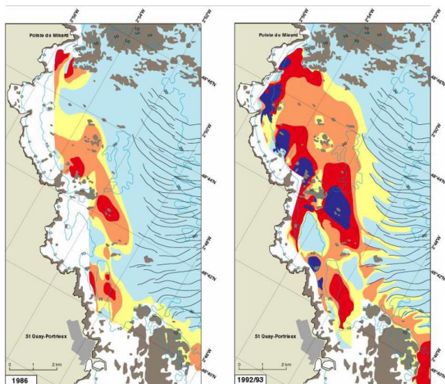
Evolution de la colonisation des fonds par la crépidule dans le secteur occidental de la baie de Saint-Brieuc entre 1986 et 1992. Source : Ifremer. REBENT
