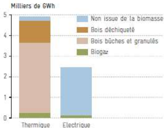
Figure 16 : Sources d'énergie dans la production énergétique totale bretonne en 2016
