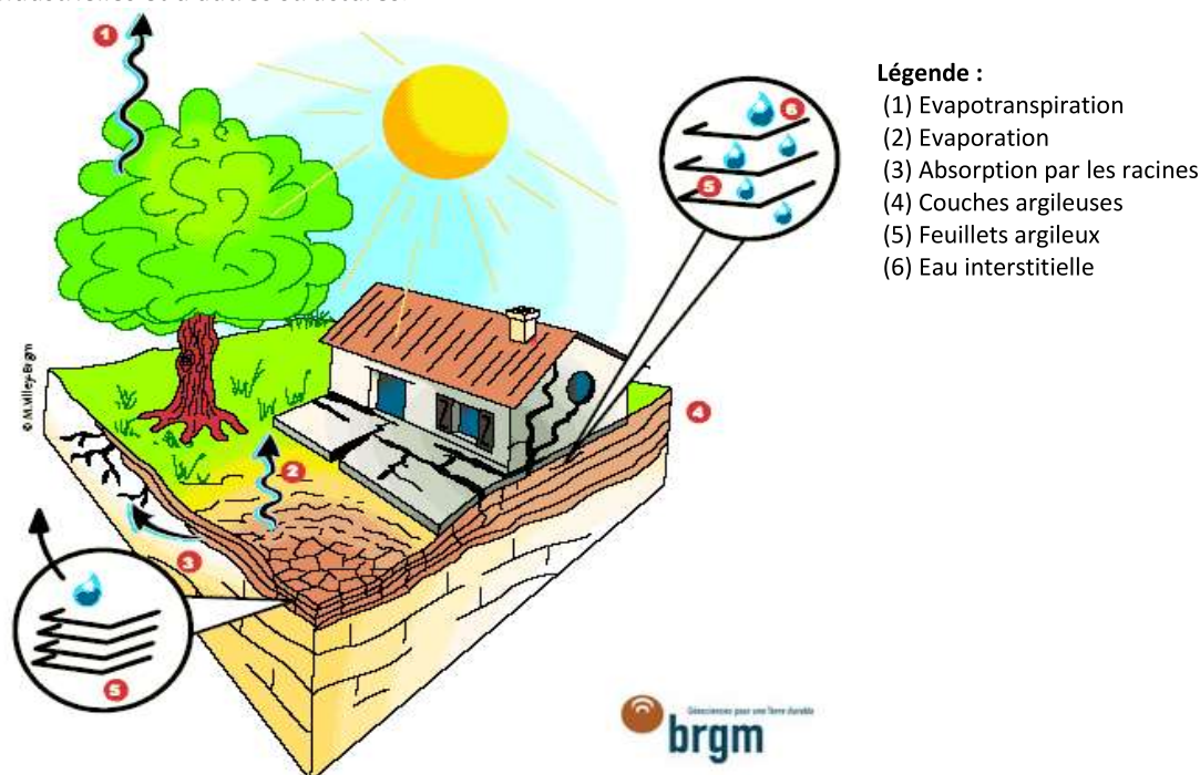
Figure 20 : Schéma du phénomène de retrait-gonflement des argiles
