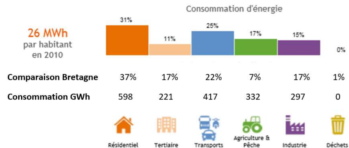
Figure 37 : Répartition des consommations d'énergie finale du territoire par secteur
