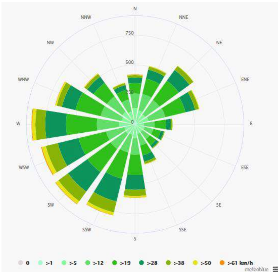
Figure 12 : Rose des vents à Guingamp exprimé en nombre d'heures par an, réalisée par le modèle de Météo Blue
