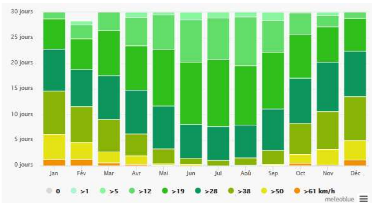
Figure 13 : Répartition de la puissance des vents par mois à Guingamp, réalisée par le modèle de Météo Blue
